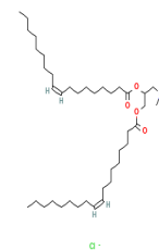
CAS Number: 132172-61-3
