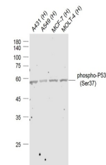
Western blot: Lane 1:A431 (Human) Cell;La...
