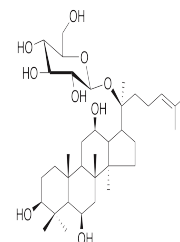
Chemical structure of Ginsenoside F1
