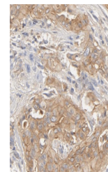
ATXN3 antibody
