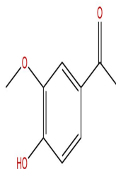
Acetovanillone
