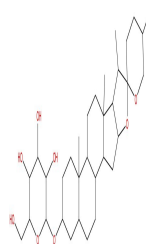
Timosaponin A1
