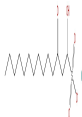
Sodium Houttuyfonate
