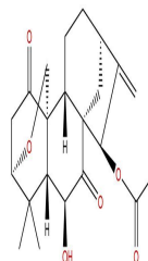
Maoecrystal A
