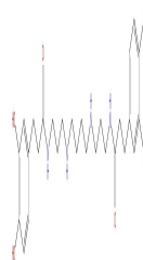
Kukoamine A
