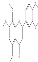
Isosinensetin
