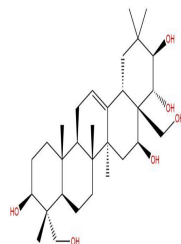
Gymnemagenin
