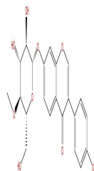
4'- methoxy- Daidzin
