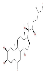
25R- Inokosterone
